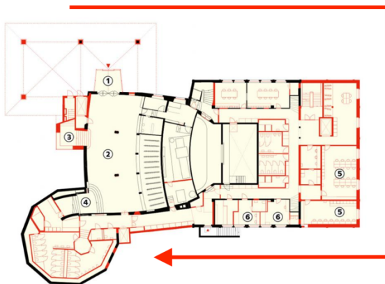
Unten: Eingangsgeschoss, Mst. 1:600. ① Eingang/Windfang ② Eingangshalle ③ Aufgang ins Boesch-Foyer (ehemals Bölsterli-Foyer) ④ Aufgang ins Sachs-Foyer ⑤ Sammelgarderoben ⑥ Einzelgarderoben
